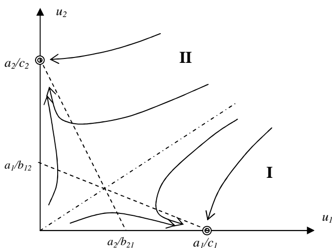
Рис.6. Динамика изменения "силы" субъектов в ходе конкурентной борьбы в системе с c_i/b_{ji} < 1 (пунктирные линии - изоклины, штрих-пунктирная линия - сепаратриса, точки - устойчивые состояния)
