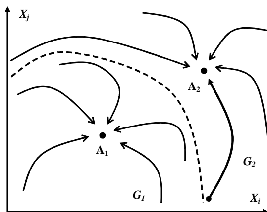
Рис.1. Типовая структура фазового пространства социальной системы с двумя устойчивыми состояниями A_1 и A_2 и соответствующими им областями притяжения G_1 и G_2 .
