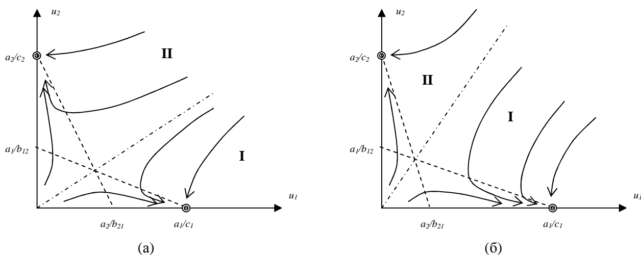
Рис.7. Изменение фазовых траекторий в обществе Восточного типа при уменьшении отношения c_1/b_{21} : (а) - начальное состояние, (б) - конечное состояние.
