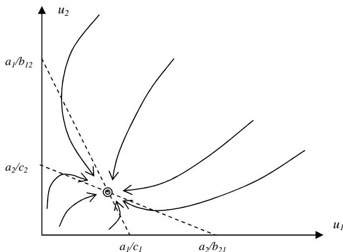
Рис.5. Динамика изменения "силы" субъектов в ходе конкурентной борьбы в системе с c_i/b_{ji} > 1 (пунктирные линии - изоклины, точка - устойчивое состояние с координатами u_{01} и u_{02} )
